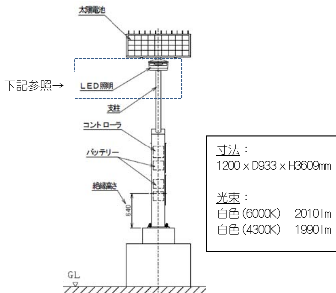
[図：ソーラー式 LED 照明の構成]
